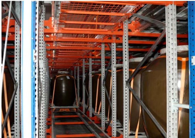
国台酒业打造的全封闭基酒管道输送系统，高效、便捷、精准。两层式立体排架存酒，每坛酒配备专属二维码，包含所有信息，提高基酒出库、入库精准管理。
